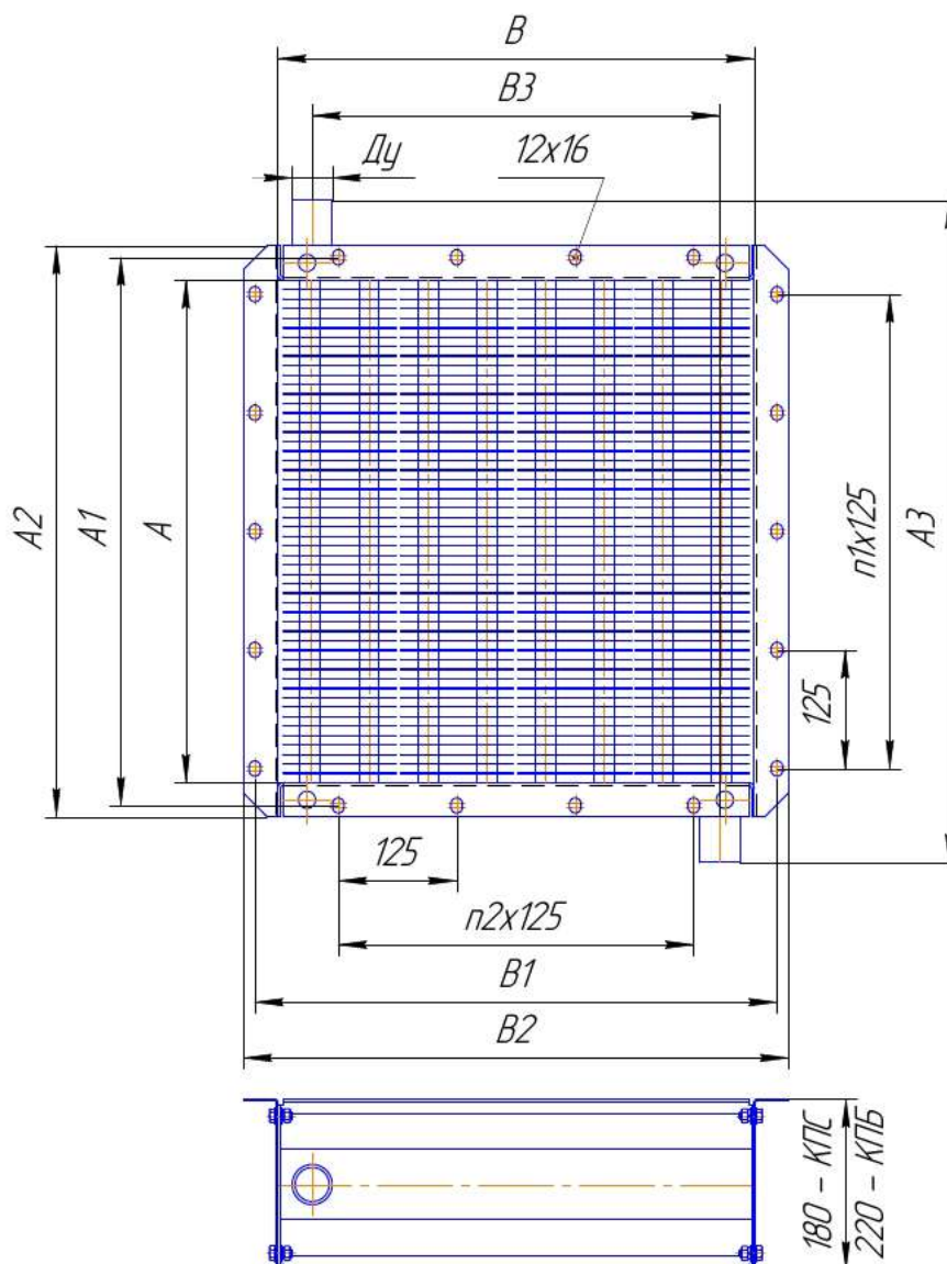
Габаритные и присоединительные размеры калориферов КПС и КПБ.
